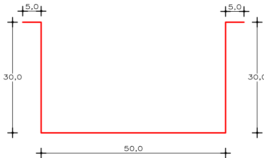
CALHA TIPO 1 SEM ESCALA CONFERIR MEDIDAS NO LOCAL, APOS A REMOÇÃO DAS TELHAS, PARA VERICAR DOBRAS.
