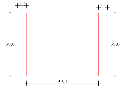
CALHA TIPO 2 SEM ESCALA CONFERIR MEDIDAS NO LOCAL, APOS A REMOÇÃO DAS TELHAS, PARA VERICAR DOBRAS.
