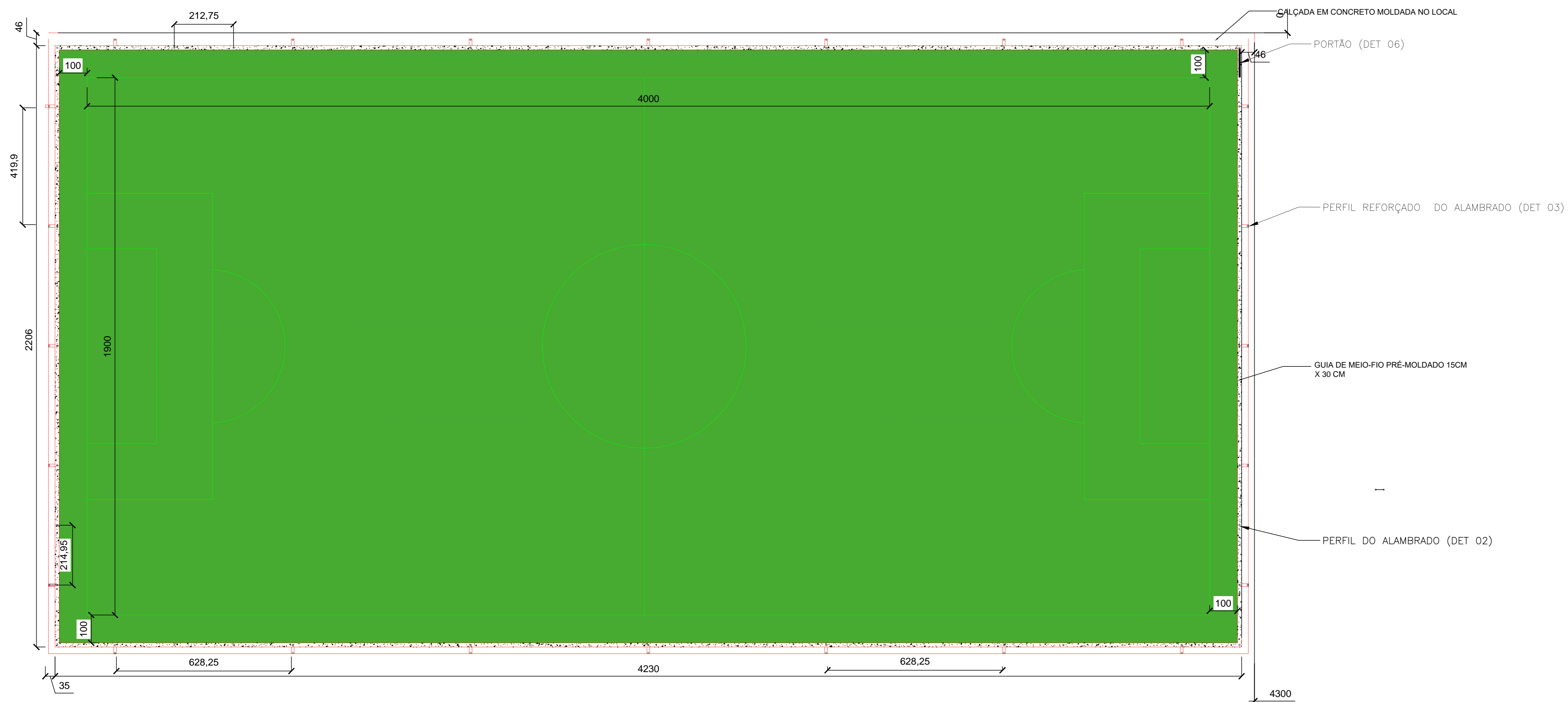
PLANTA BAIXA CAMPO SOCIETY SEM ESCALA MEDIDAS EM CENTIMENTOS
