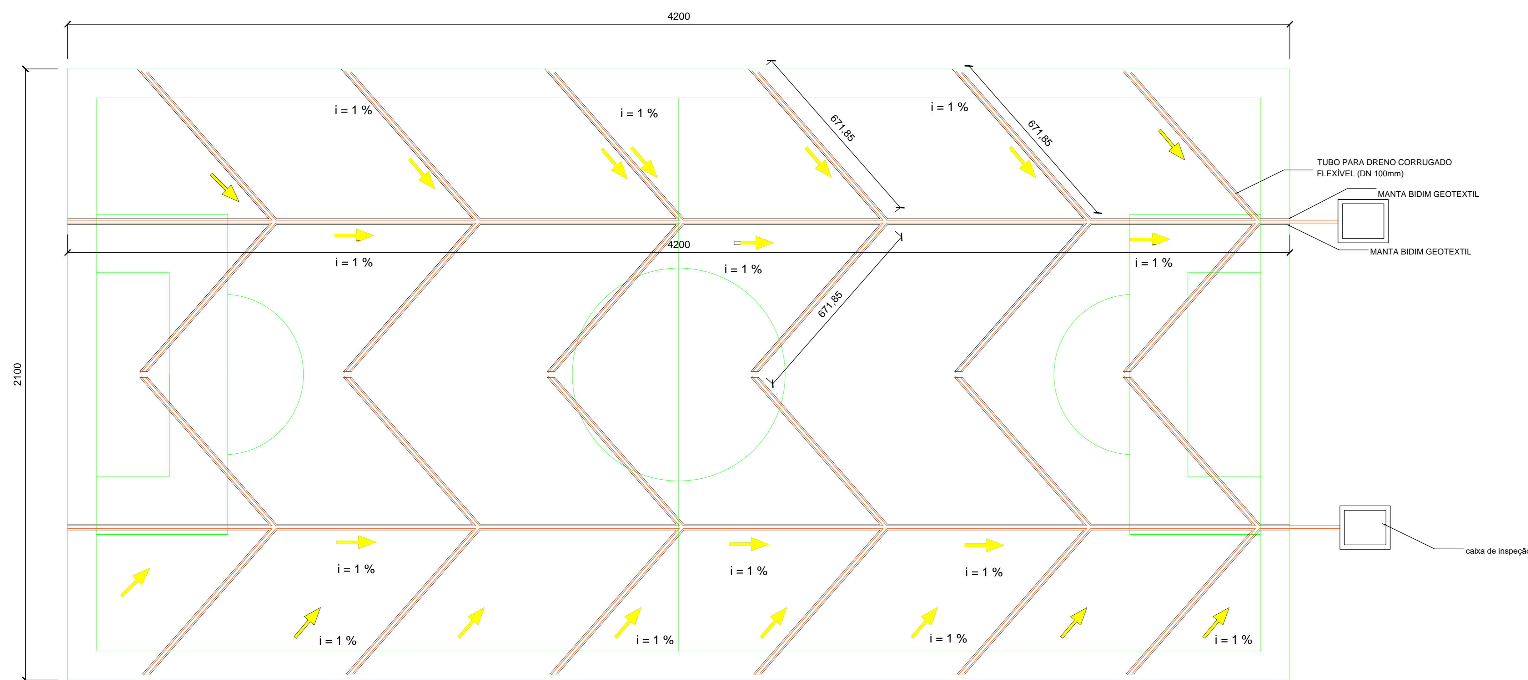
DETALHAMENTO DO DRENO CAMPO SOCIETY SEM ESCALA MEDIDAS EM CENTIMENTOS
