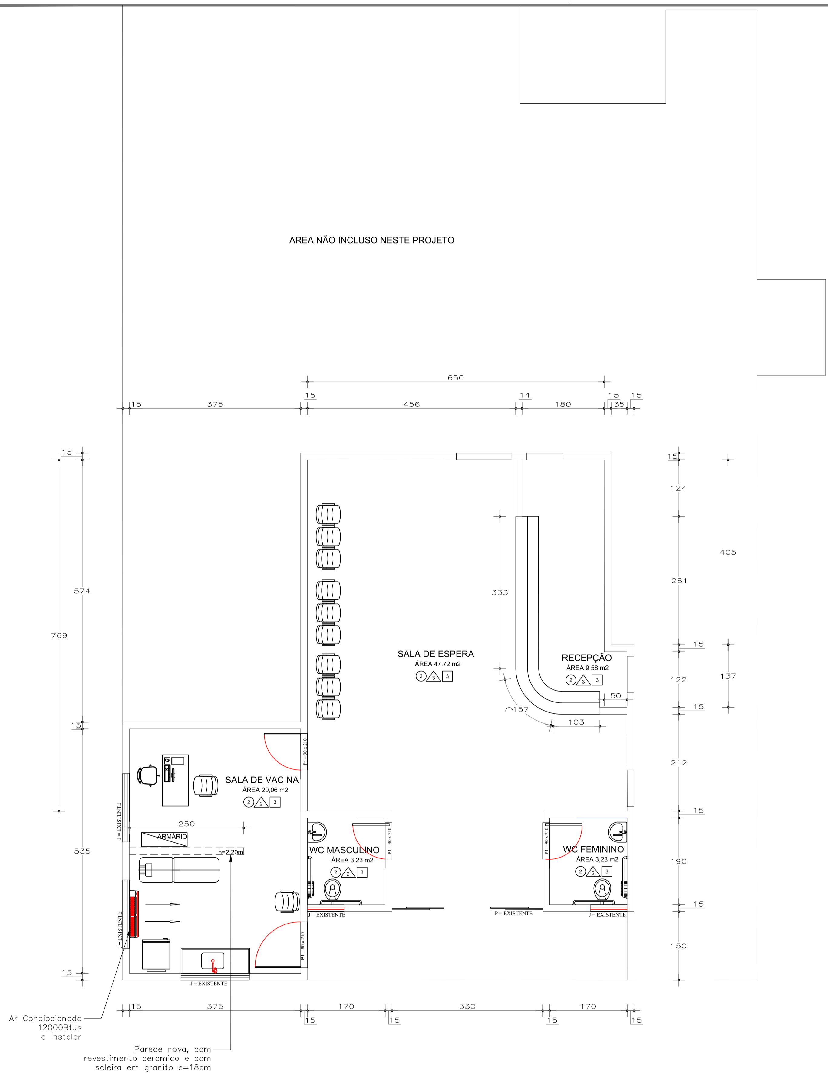
PLANTA ARQUITETONICO – AREA DE VACINAÇÃO ESCALA 1 : 50 AREA DE VACINAÇÃO 93,45M2
