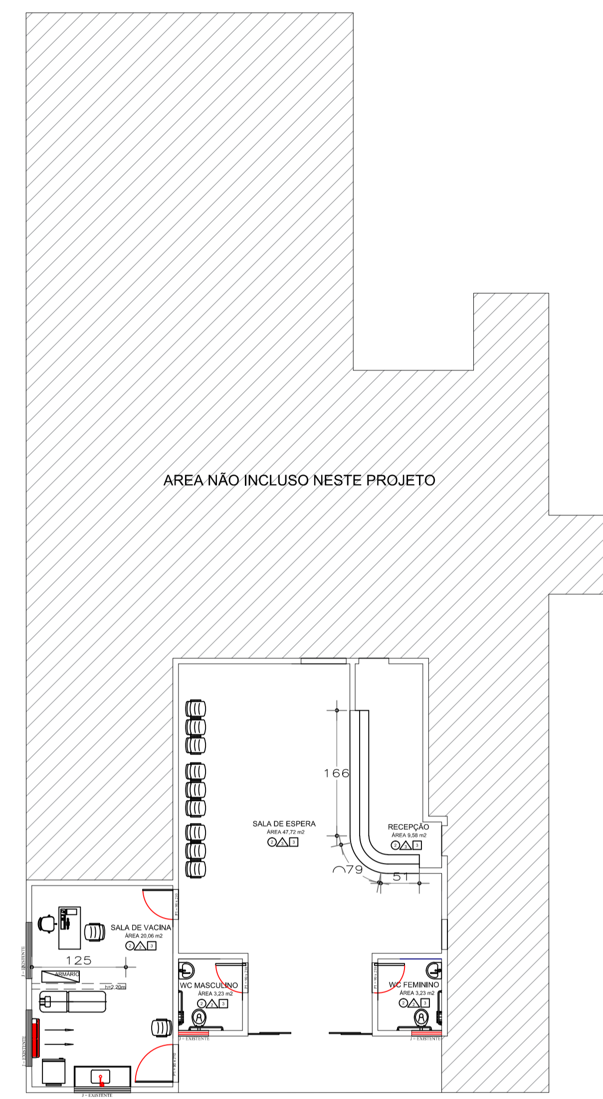
PLANTA ARQUITETONICO – AREA DE VACINAÇÃO ESCALA 1 : 100 AREA DE VACINAÇÃO 93,45M2
